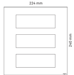
18 Module Plate
